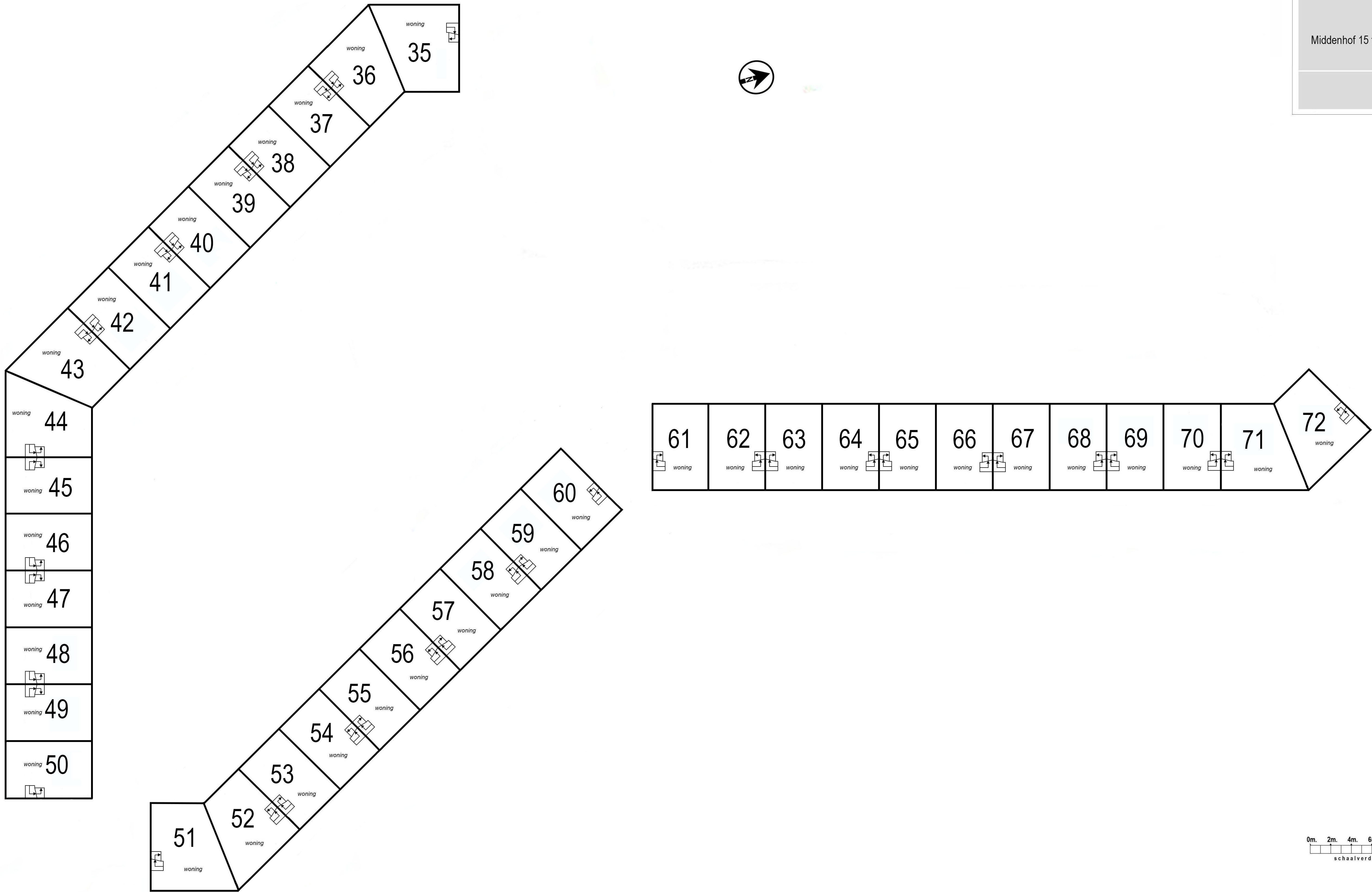
2e Verdieping 1:200
